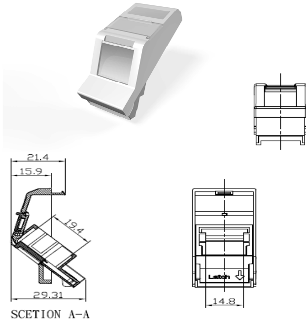
SCETION A-A
